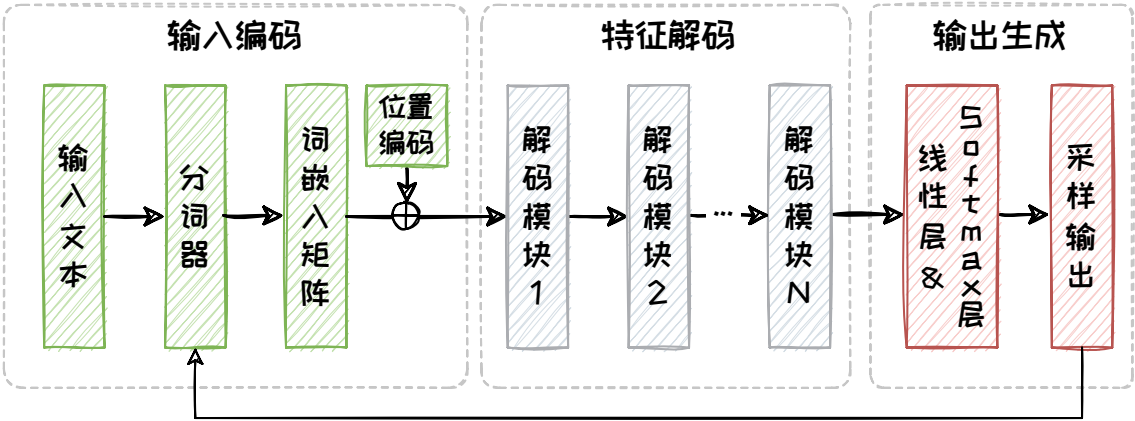
图 2.5: Decoder-only 架构。
