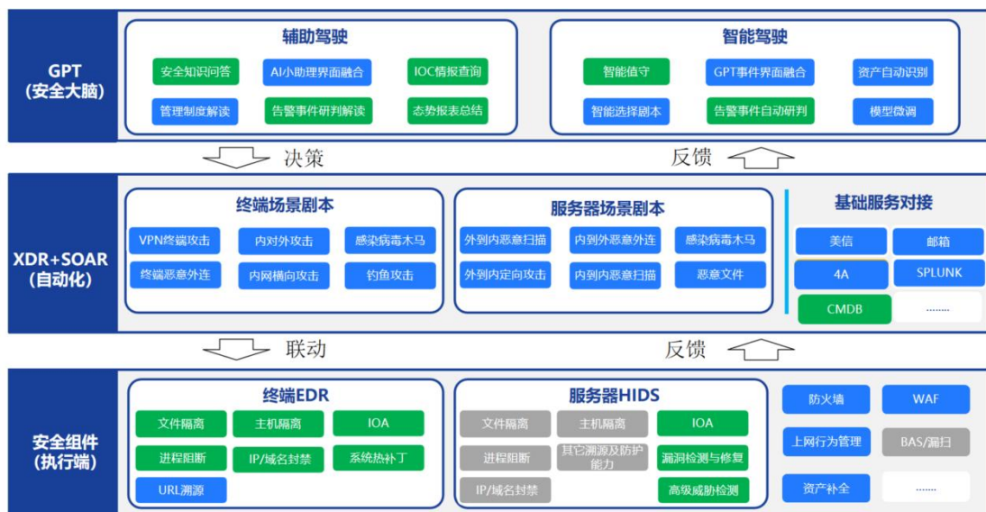
图 15 智能安全运营技术架构图
