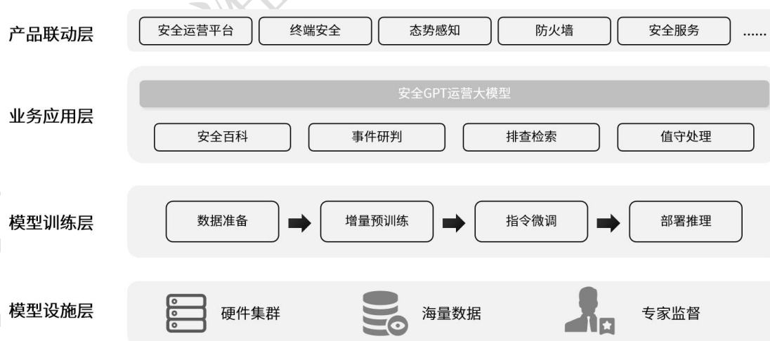
图 13 安全运营平台技术架构
