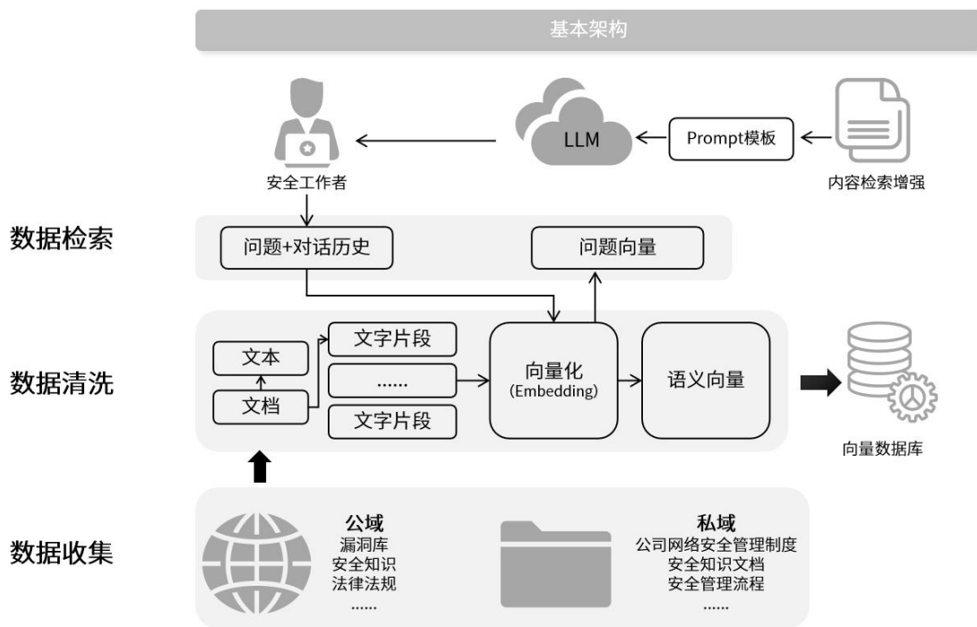
图 14 “小微”基本架构图
